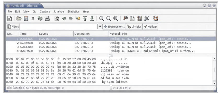
Paquetes de Syslog capturados con Ethereal
